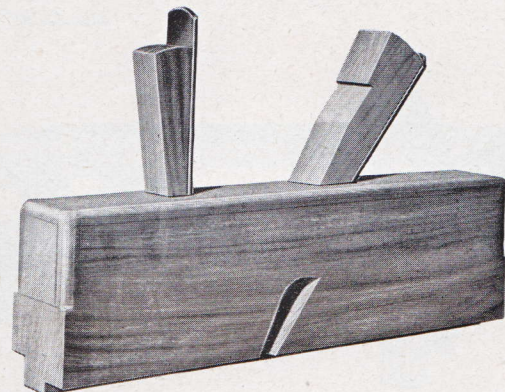
N° 127 ENTAILLE DE PERSIENNES ET DE TABLETTES
